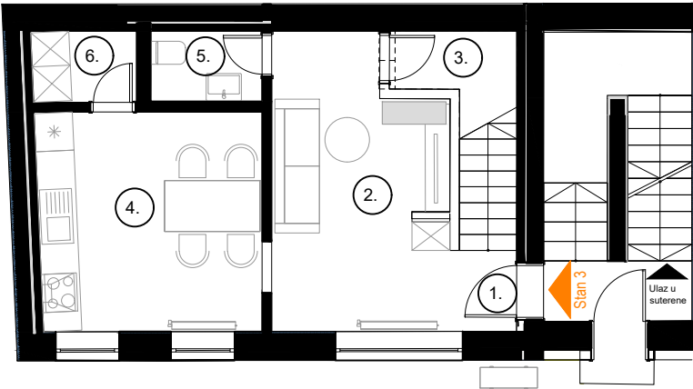
Tlocrt prizemlja
